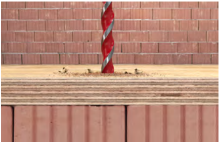
Bohren der Materialkombination Holz und Mauerwerk
